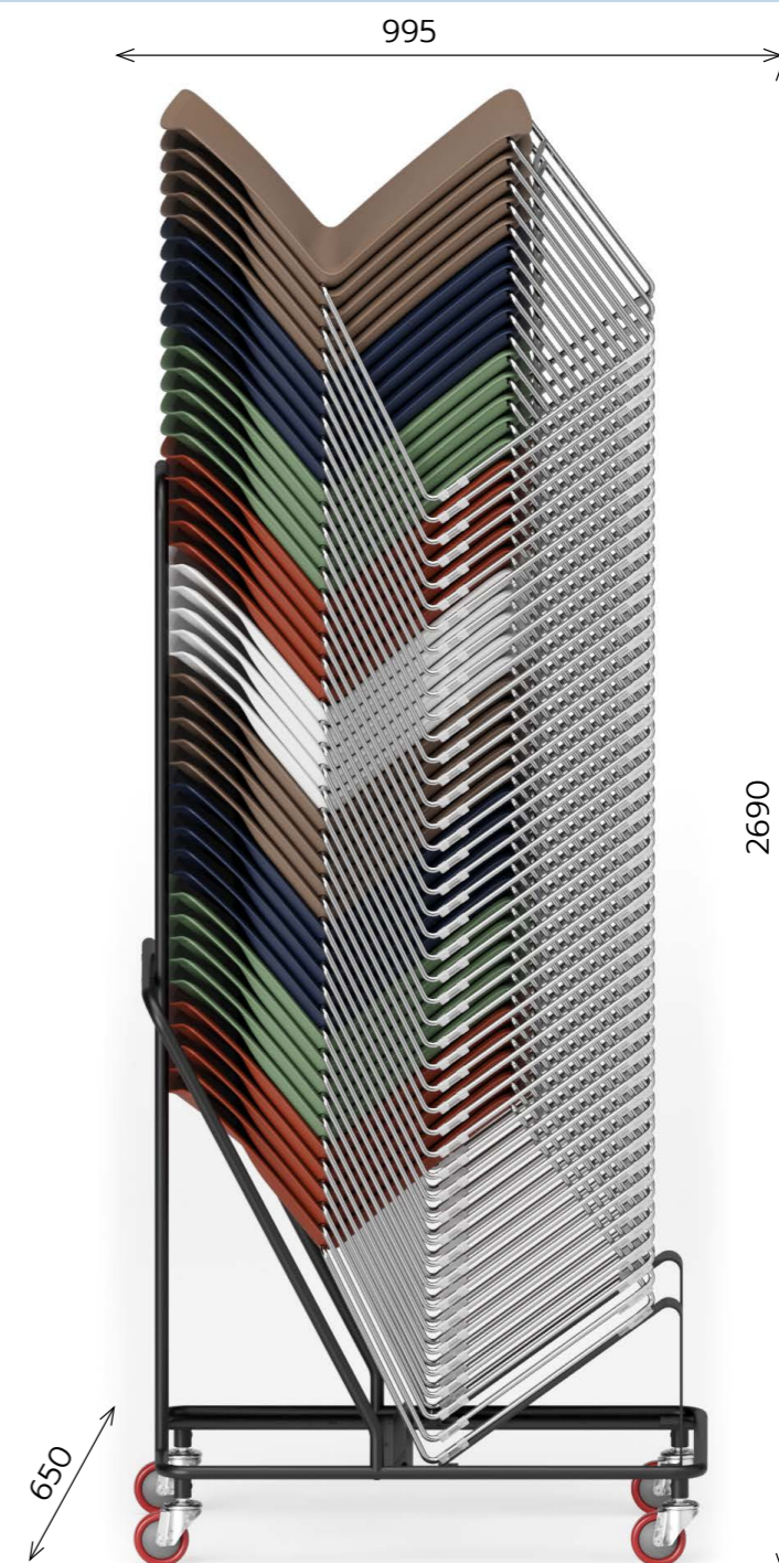
Impilabilità su carrello con inclinazione a 45°: fino a 45 per versione con telaio slitta, fino a 30 per versione con telaio 4 gambe. Stackability on trolley with 45° inclination: up to 45 for version with sled frame, up to 30 for version with 4-leg frame.
